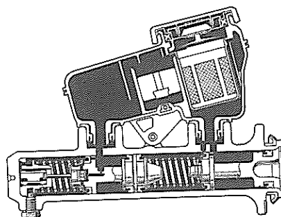
ABS装着車(除2L-TE)
