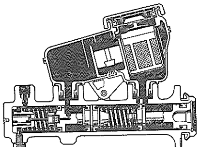
ABS装着車(2L-TE)
